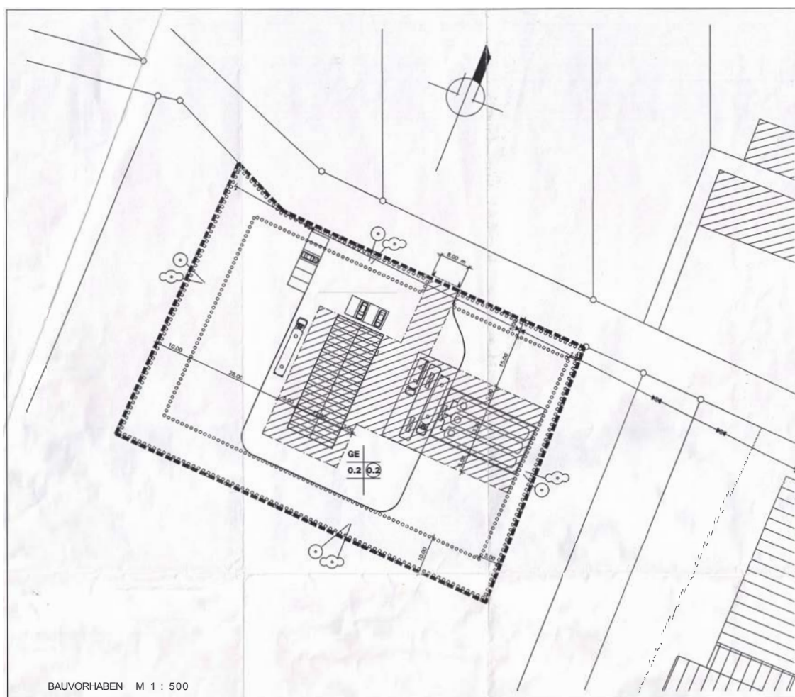
ABBILDUNG 5 PLANZEICHNUNG 1993 - ÜBERBLICK
